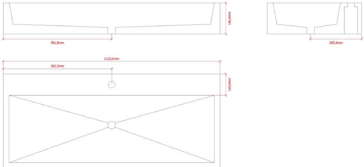
Waschbecken XL mit 3 cm Rand und 11 cm Bank + mittige Bohrung für Armatur Außenmaße ca. 112,5 x 49 x 16 cm ( BxTxH )
